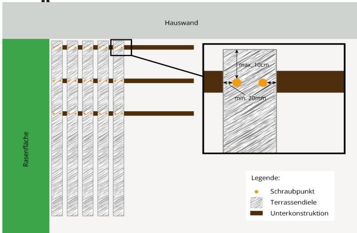
Verlegung über die volle Länge
